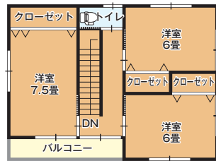
2階 平面図
